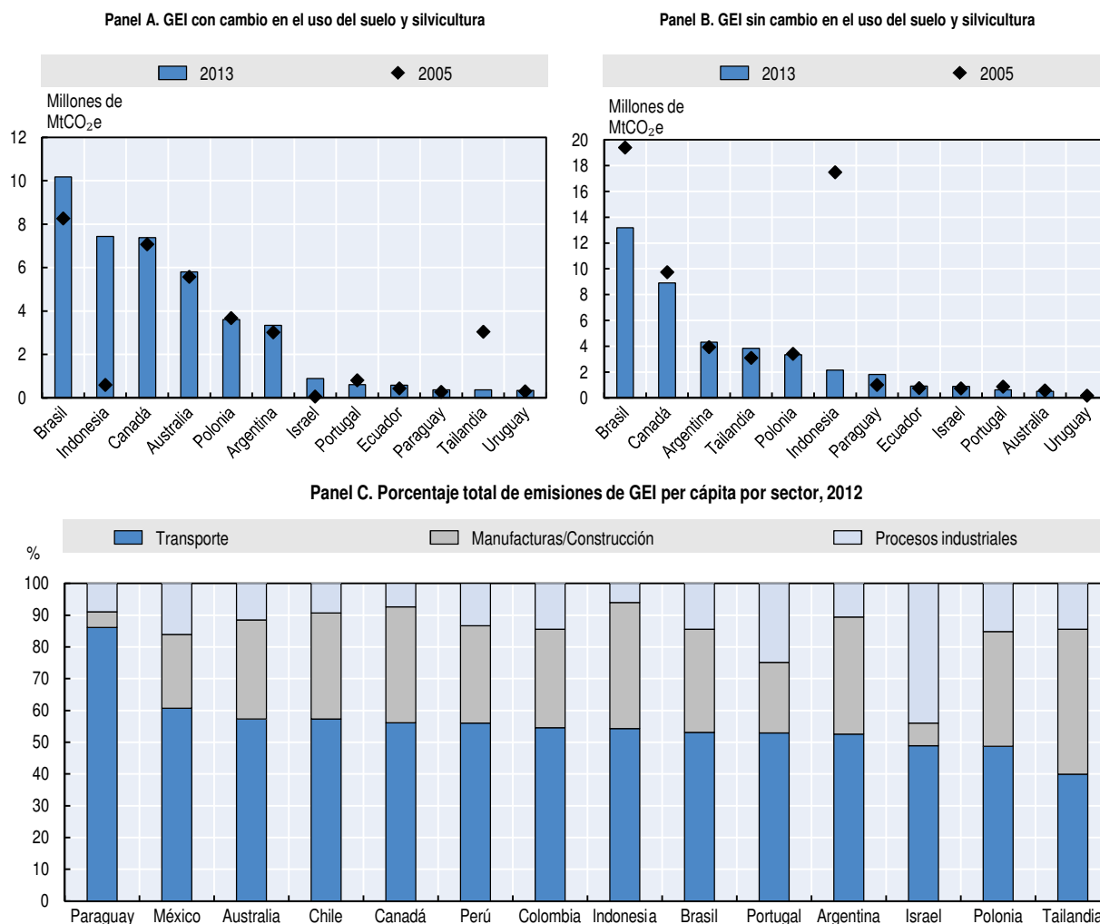
Gráfico 4.9. Emisiones totales de gases de efecto invernadero (GEI) con y sin cambios en el uso del suelo y silvicultura (toneladas métricas de dióxido de carbono equivalente, Mt CO 2 e)
