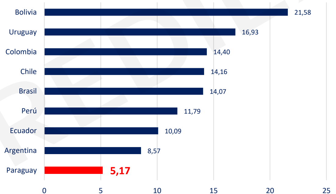
COÛT EN CENTS USD PAR KWH (2019) TARIF COMMERCIAL À PARTIR DE 50000 KW / MOIS
